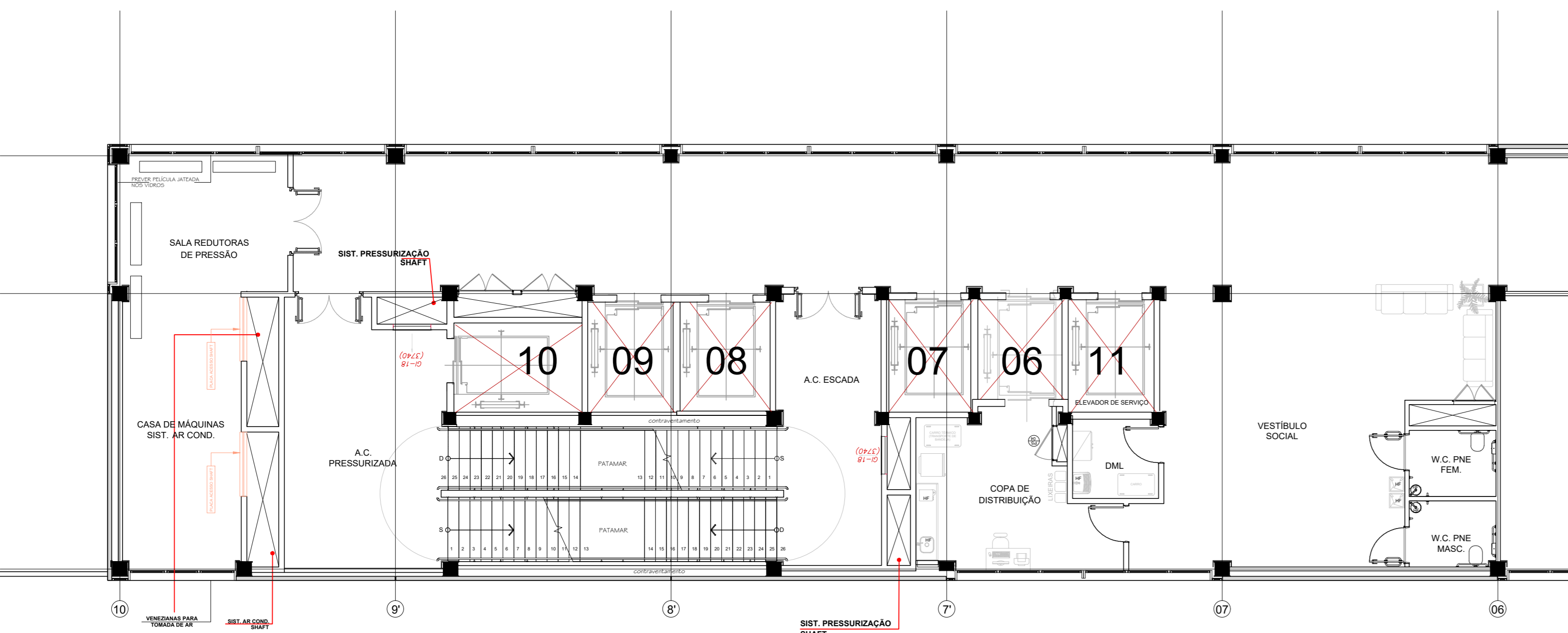
PLANTA 1º PAVIMENTO (ALA A)
